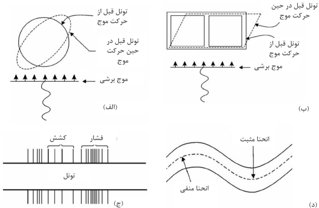
شکل ۴-۱- مودهای تغییر شکلی تونل تحت انتشار امواج، (الف) بیضوی در تونل با مقطع دایره‌ای، (ب) اعوجاجی در تونل با مقطع مستطیلی، (ج) محوری، (د) انحنایی
